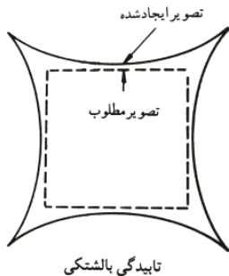
تصویر ۵: خطای بالشتکی، (لنگفورد، ۱۳۹۱: ۶۶)
