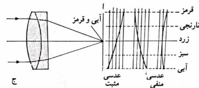
تصویر ۹: خطای رنگی، (جعفریان، ۱۳۷۶: ۱۶۹)
