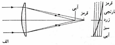
تصویر ۷: خطای رنگی، (جعفریان، ۱۳۷۶: ۱۶۹)
