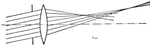
تصویر ۴: ب. ایجاد کما به دلیل تفاوت شکست پرتوهایی که به طور مایل به عدسی می‌تابند، (جعفریان، ۱۳۷۶: ۱۷۳)
