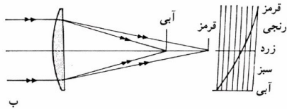
تصویر ۸: خطای رنگی، (جعفریان، ۱۳۷۶: ۱۶۹)
